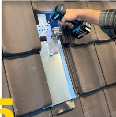
Dachhaken montieren
